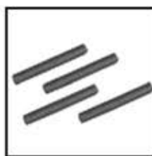
DOWEL PIN (D2m6 X 14) Ref : AVZS-05006
