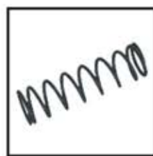
PRESSURE SPRING Ø1,4 / Ø11,9 X 4 Ref : 4FA-0008
